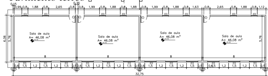
PLANTA BAIXA TÉRREO
