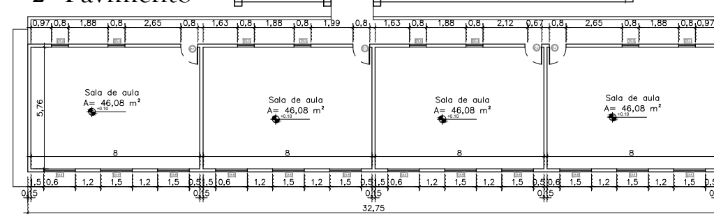
PLANTA BAIXA 2º PAVIMENTO
